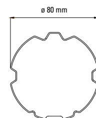
Adattatore per tubo zf 80
